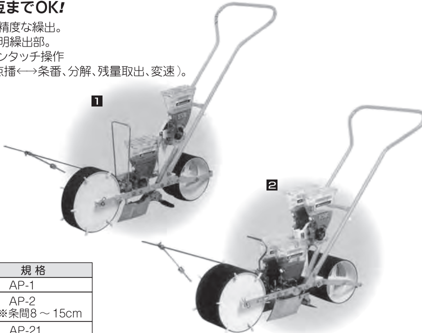
※写真は、オプションの農薬散布装置、条間マーカ付です。
